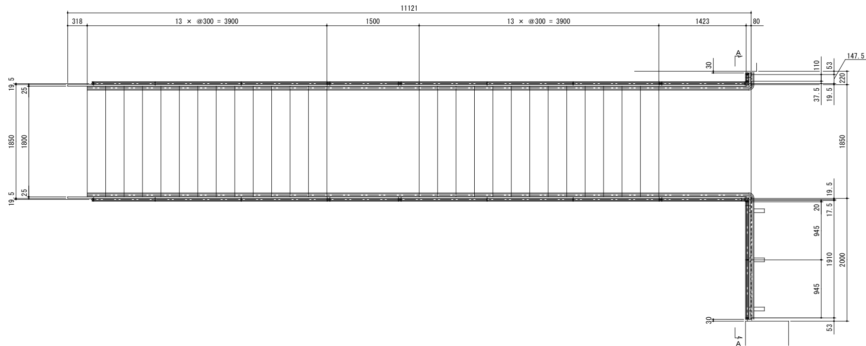
側面図 S = 1 / 30
