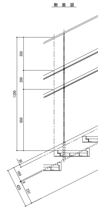
取付詳細図 S = 1 / 10
