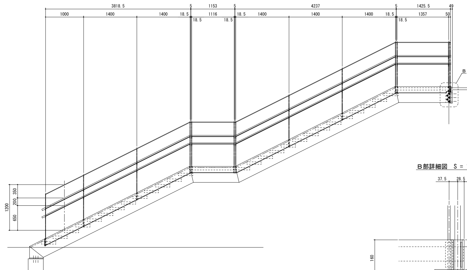
側面図 S = 1 / 30
