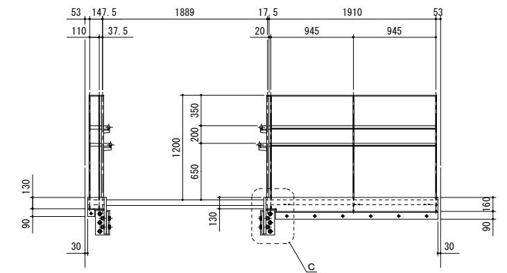
取付詳細図 S = 1 / 10
