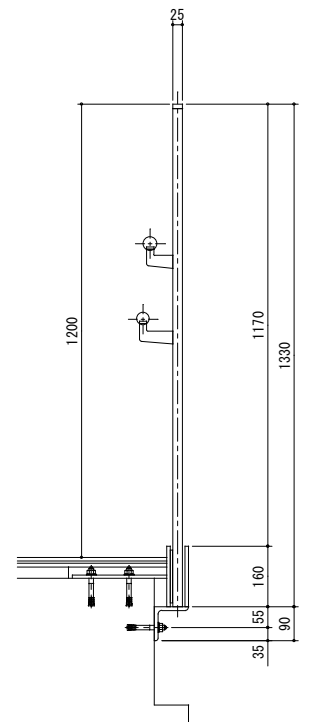
擁壁取合部
