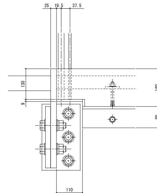
C部詳細図 S = 1 / 5
