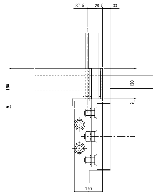
B部詳細図 S = 1 / 5
