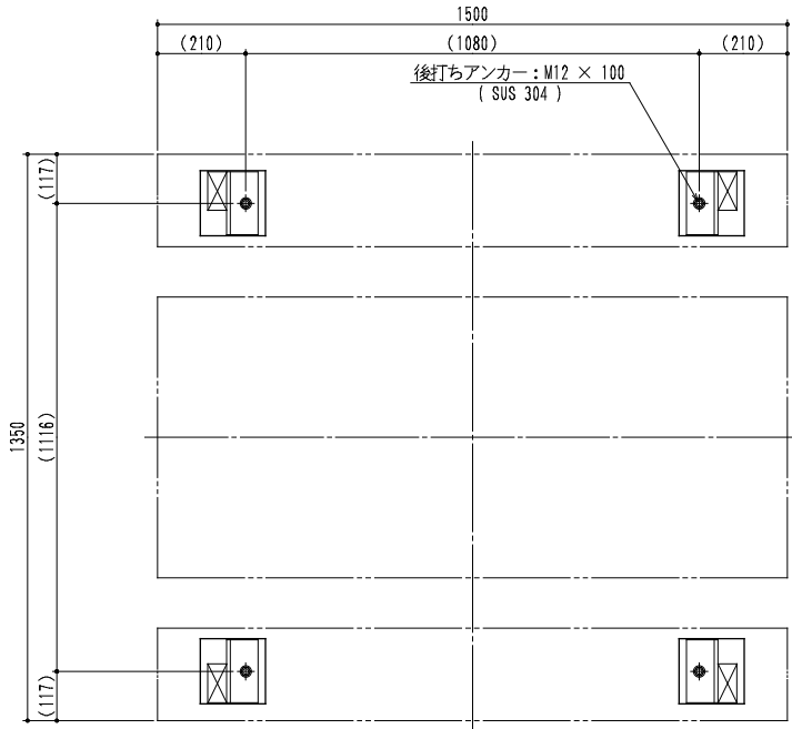
平面アンカー図 S = 1/10
