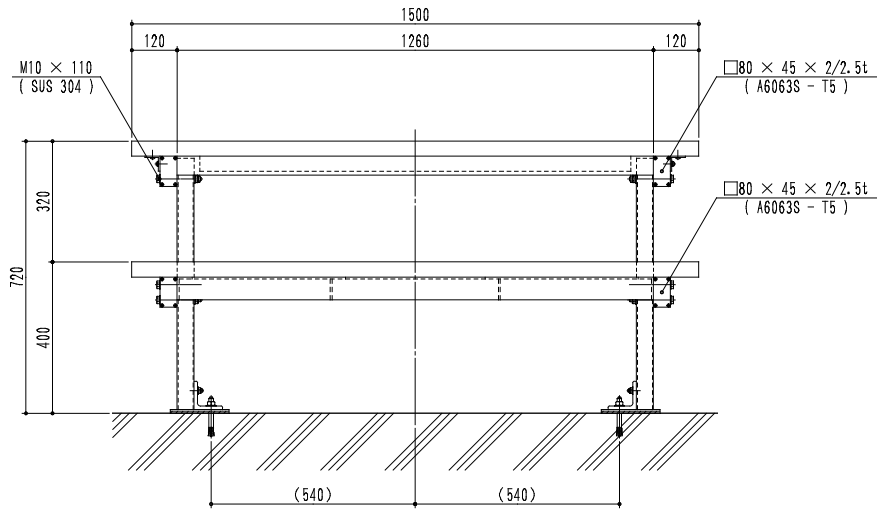
正 面 図 S = 1/10
