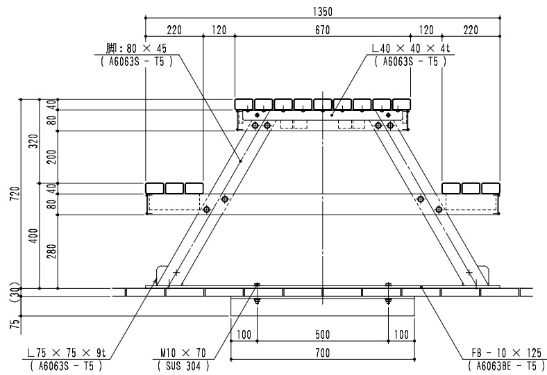
側 面 図 S = 1/10
