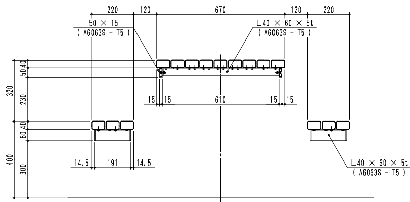
断 面 図 S = 1/10 ( A - A 断 面 )
