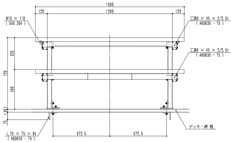
正 面 図 S = 1/10
