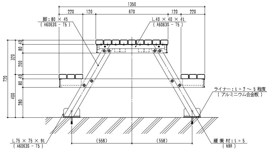
側 面 図 S = 1/10
