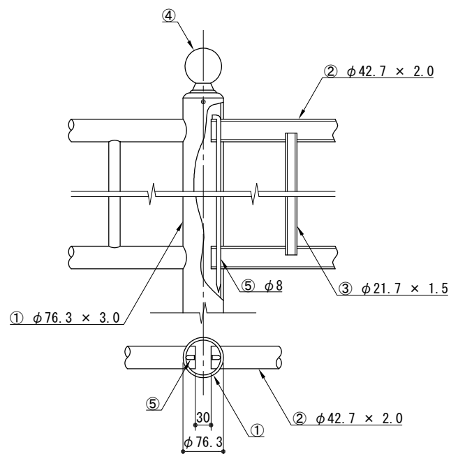
取付詳細図
