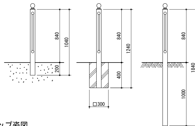
キャップ姿図
