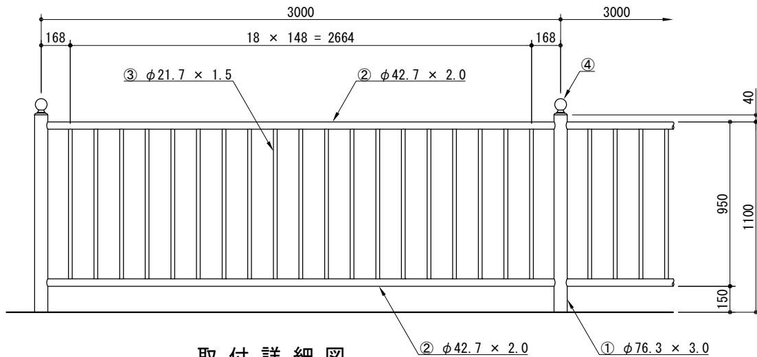
取付詳細図
