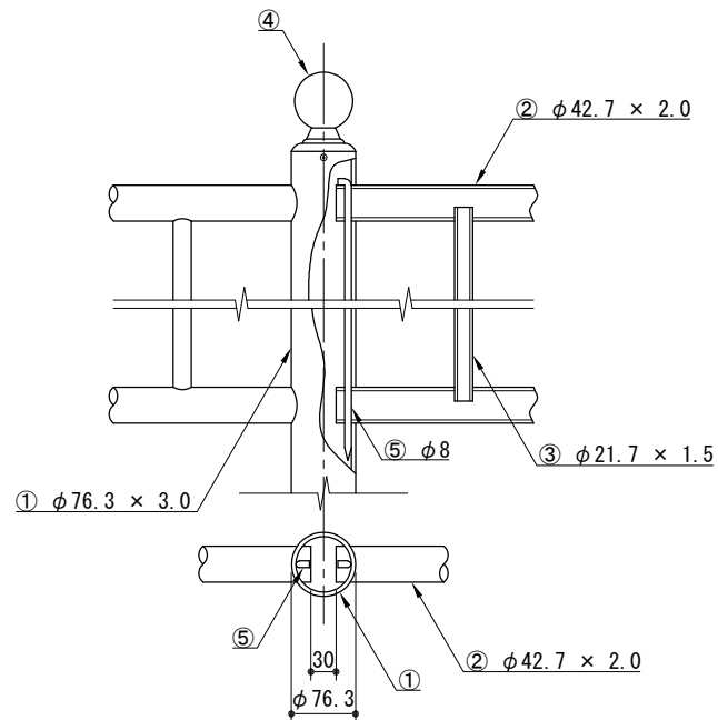
取付詳細図
