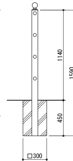
独立基礎式 (UP7-411C)
