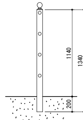
連続基礎式 (UP7-411W)
