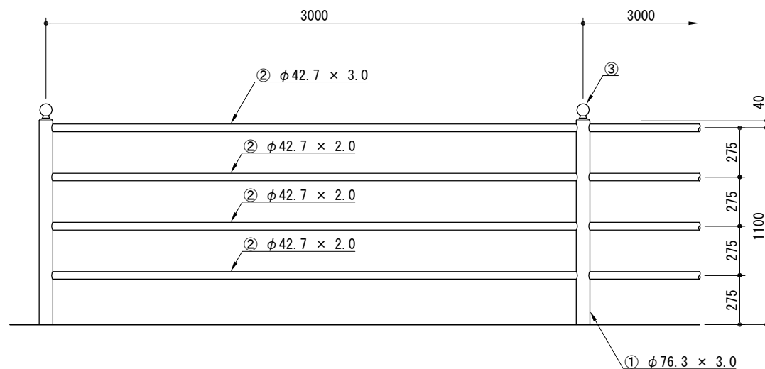
取付詳細図
