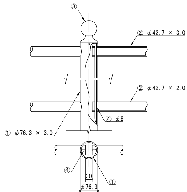
取付詳細図
