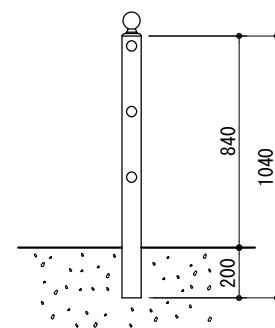
連続基礎式 (UP7 - 308W)
