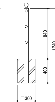
独立基礎式 (UP7 - 308C)
