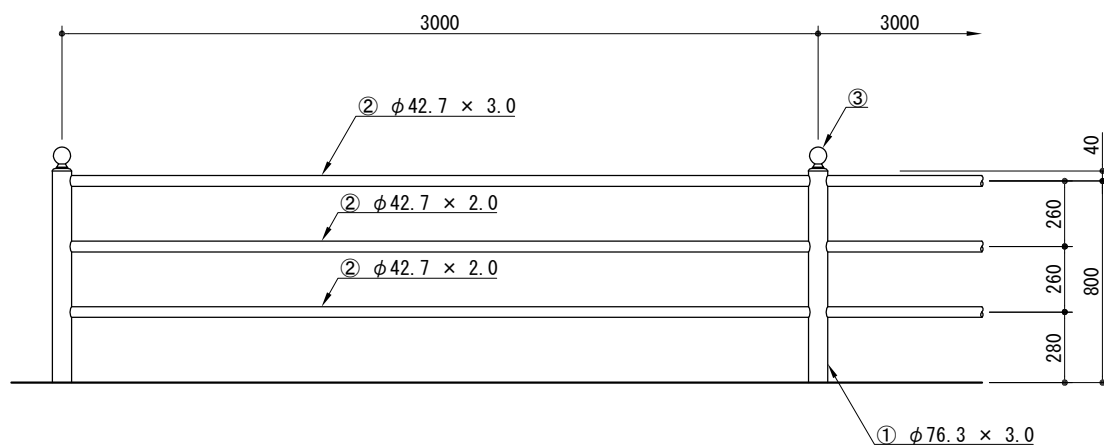
取付詳細図
