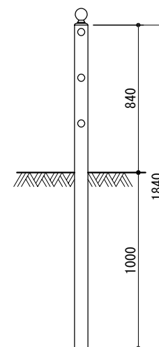
土中式 (UP7 - 308E)
