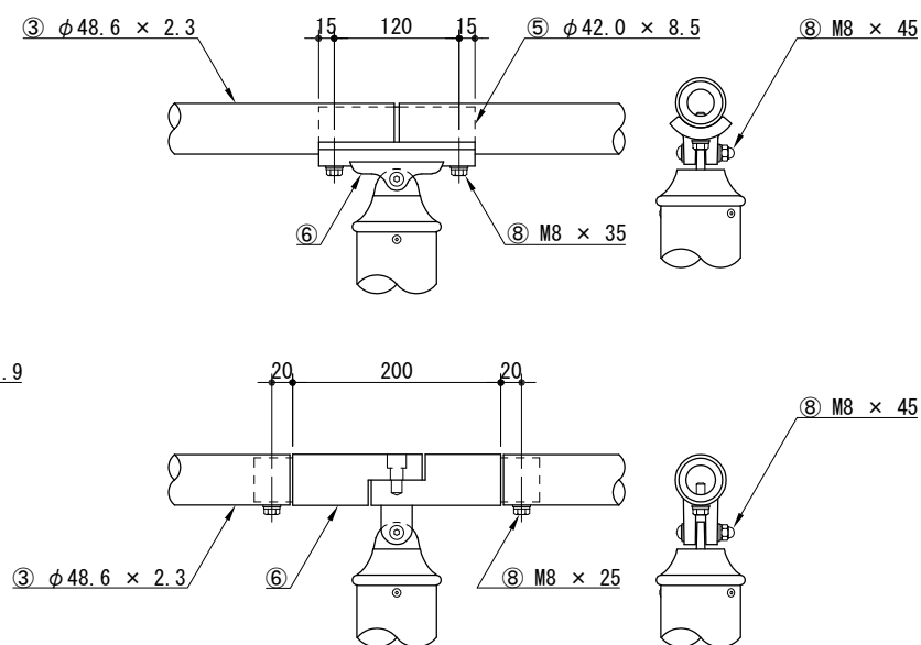
T金具詳細図
