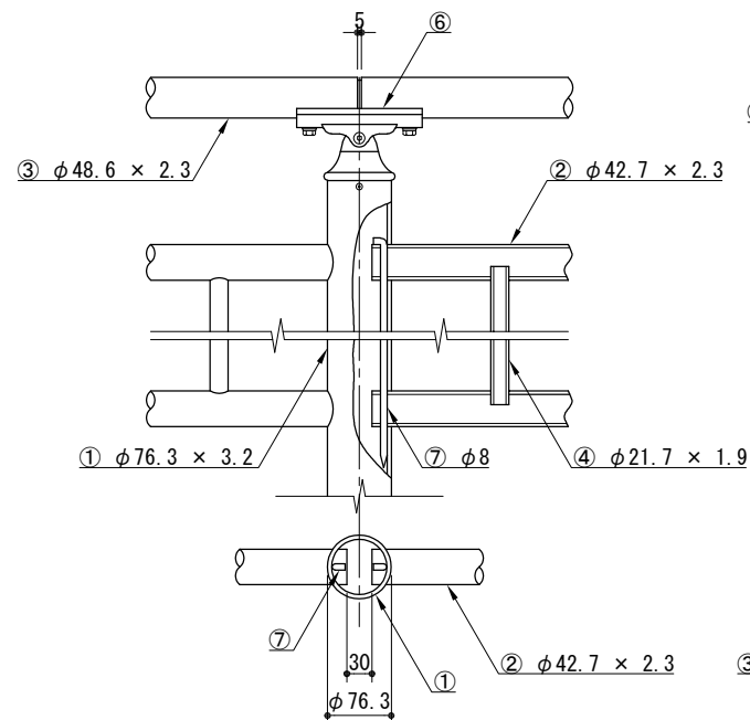
取付詳細図
