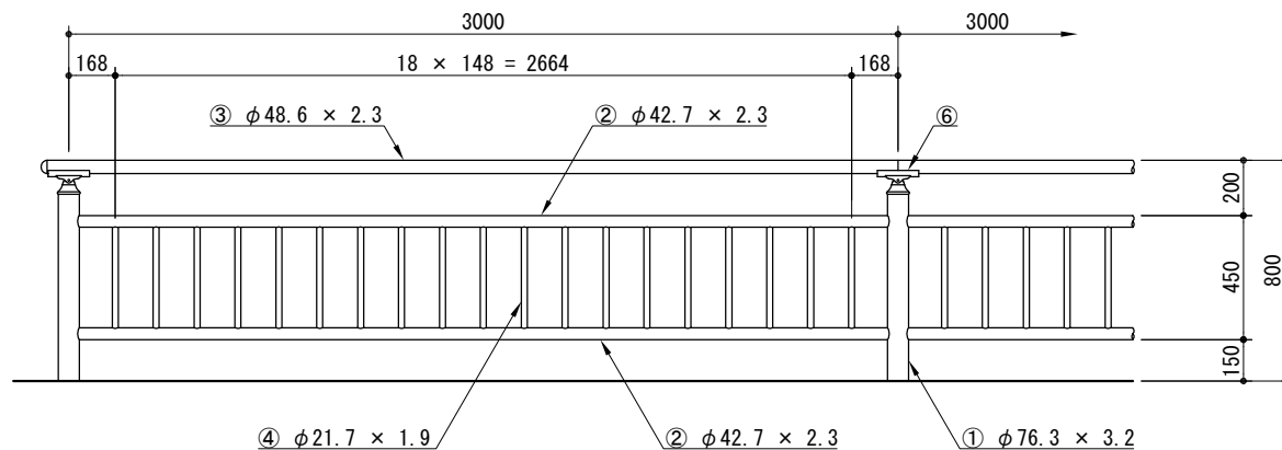
取付詳細図
