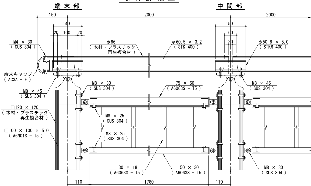
取 付 詳 細 図
