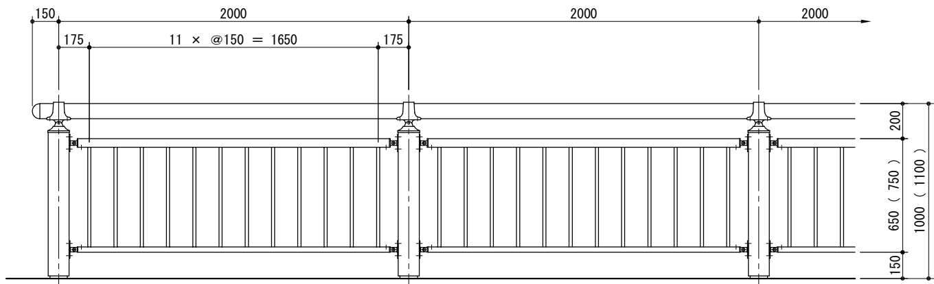
取 付 詳 細 図
