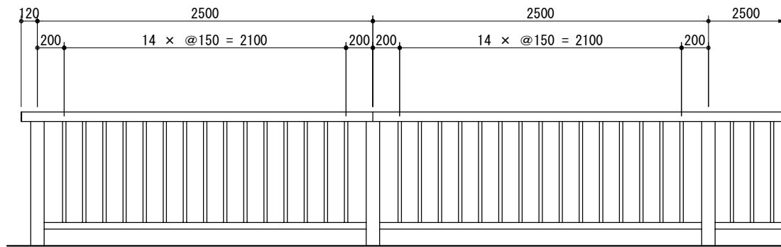
取付詳細図
