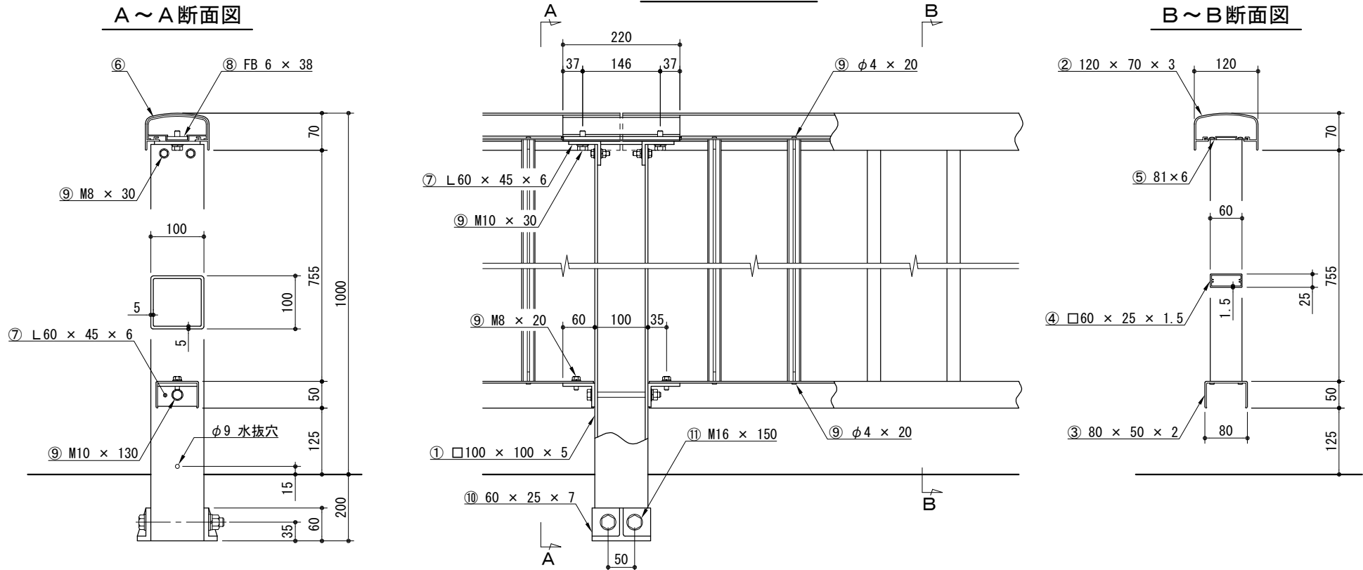
取付詳細図
