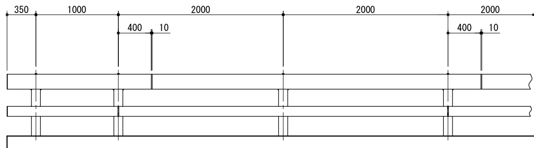
正面図
