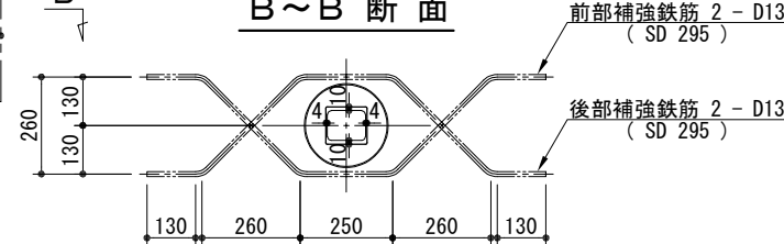
B～B 断面
