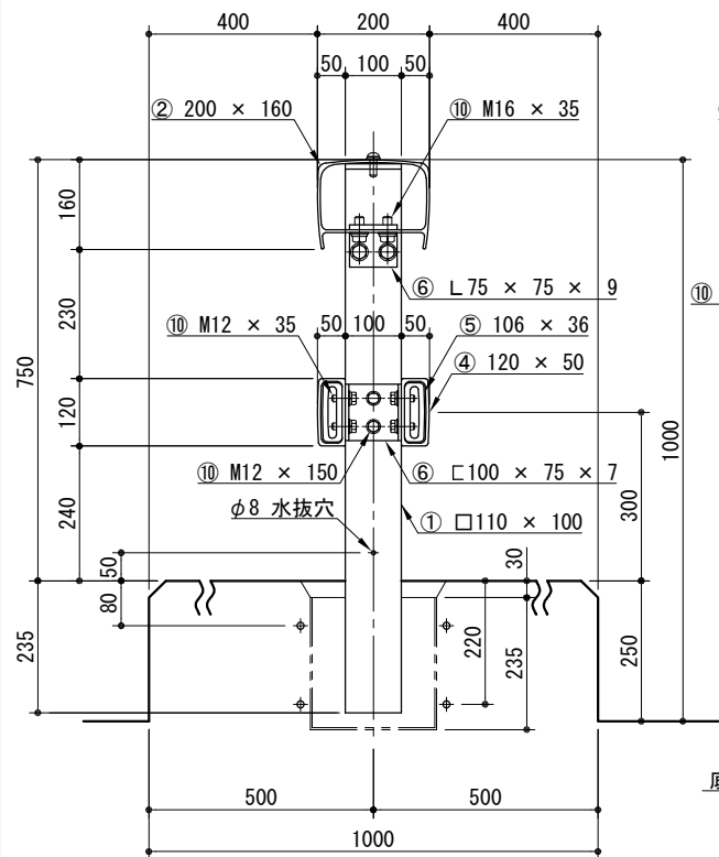
取付詳細図
