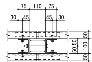
C～C 断面
