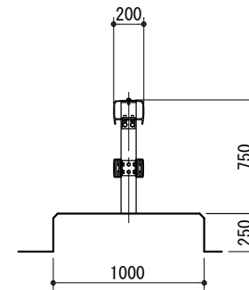
端 部
