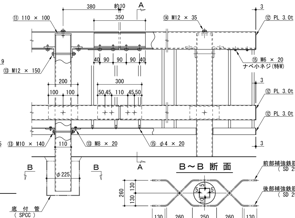
繼 手 部
