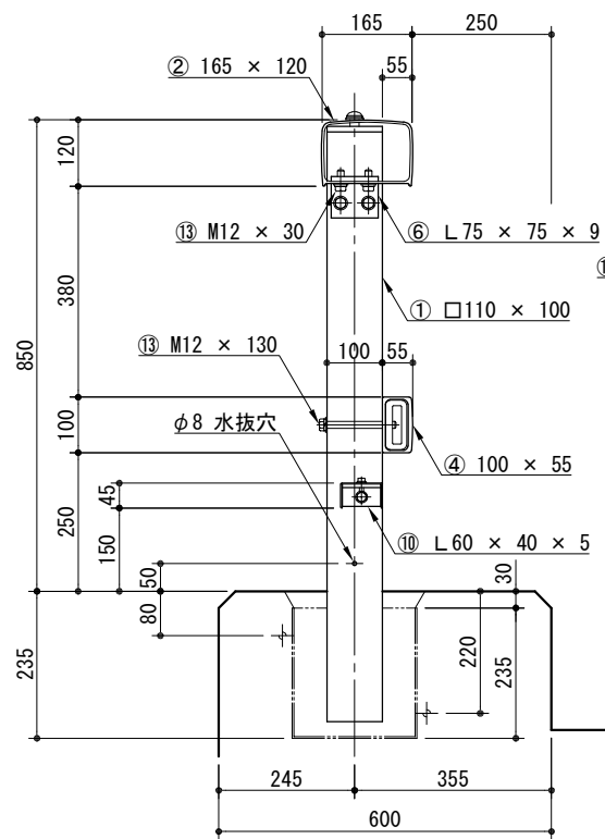
取 付 詳 細 図
