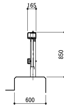
側 面 図
