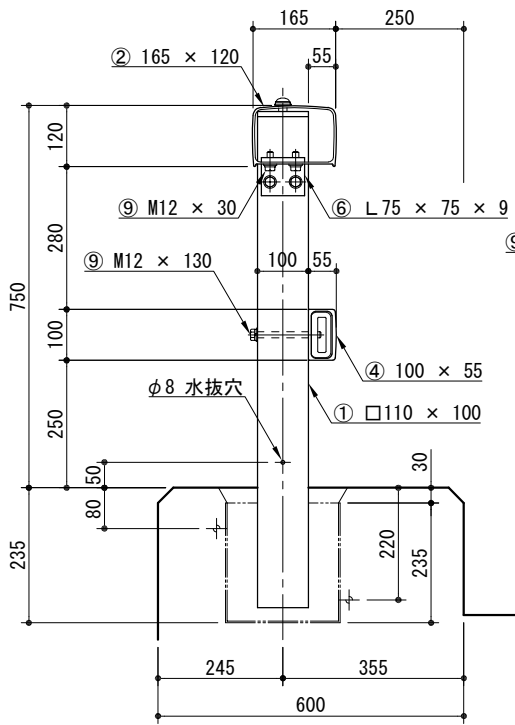
取 付 詳 細 図
