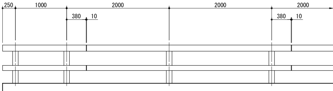
正 面 図
