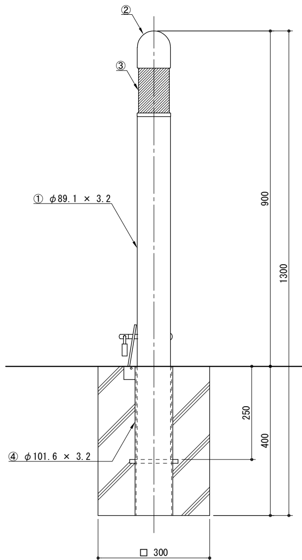
立面図
