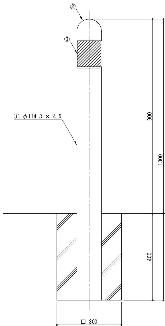
立面図
