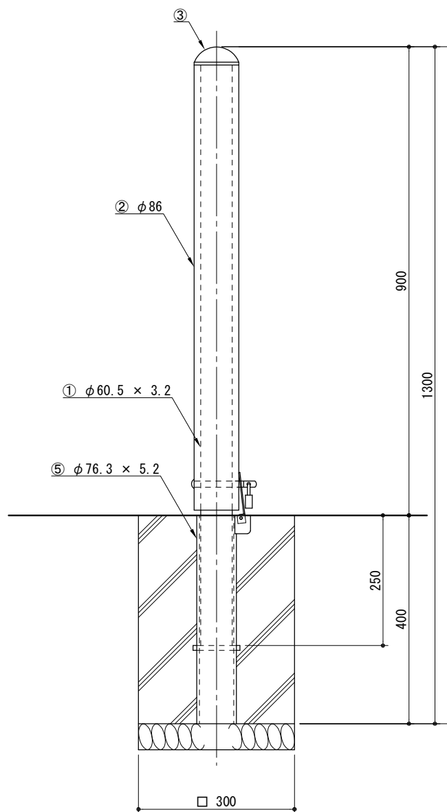
立面図
