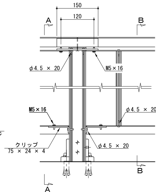
取付詳細図
