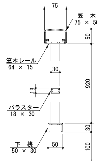
B～B断面図
