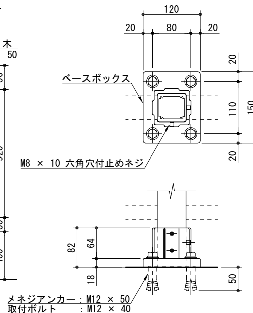
ベース部詳細図
