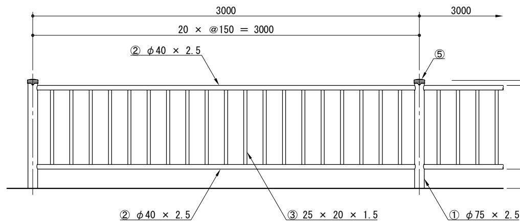
正面図
