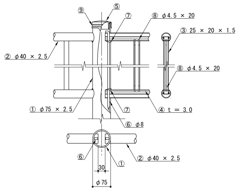
取付詳細図
