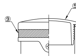
キャップ詳細図
