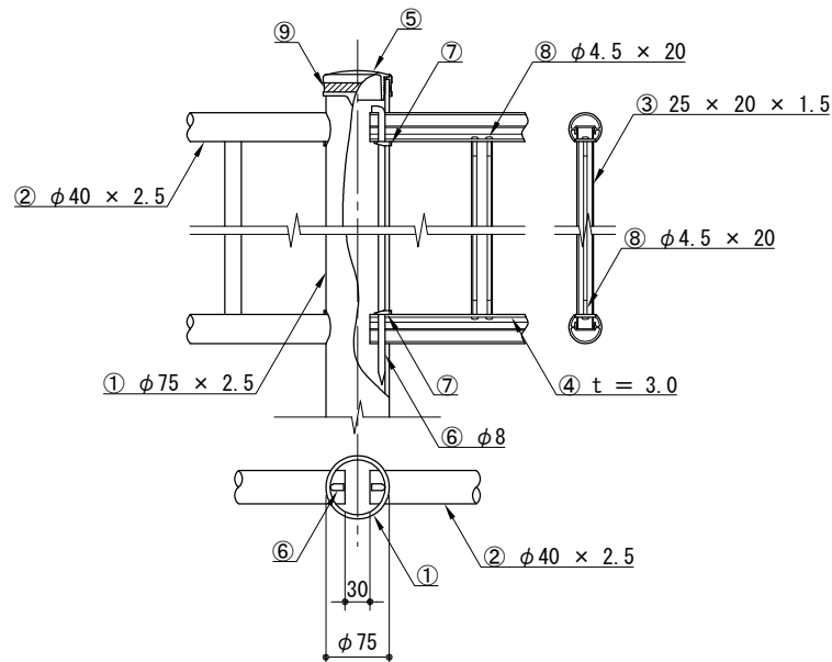
取付詳細図
