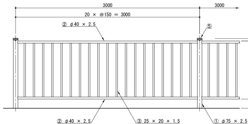
正面図
