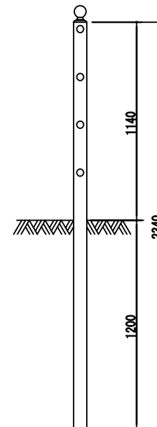
土中式 ( P7 - 411E )
