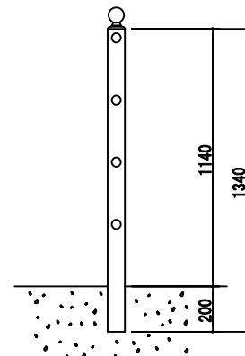
連続基礎式 ( P7 - 411W )
