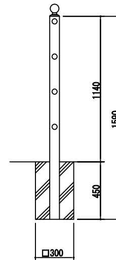
独立基礎式 ( P7 - 411C )
