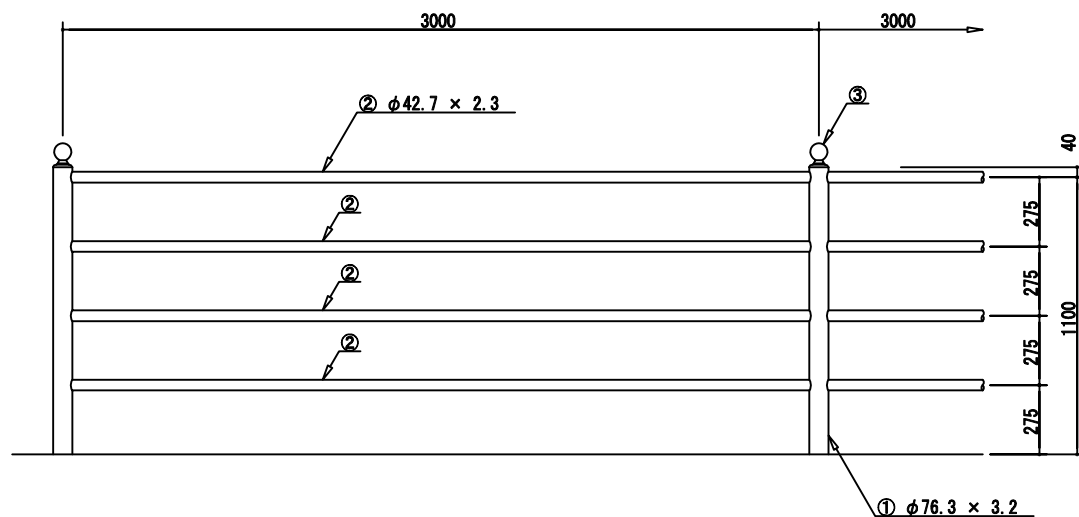
取付詳細図
