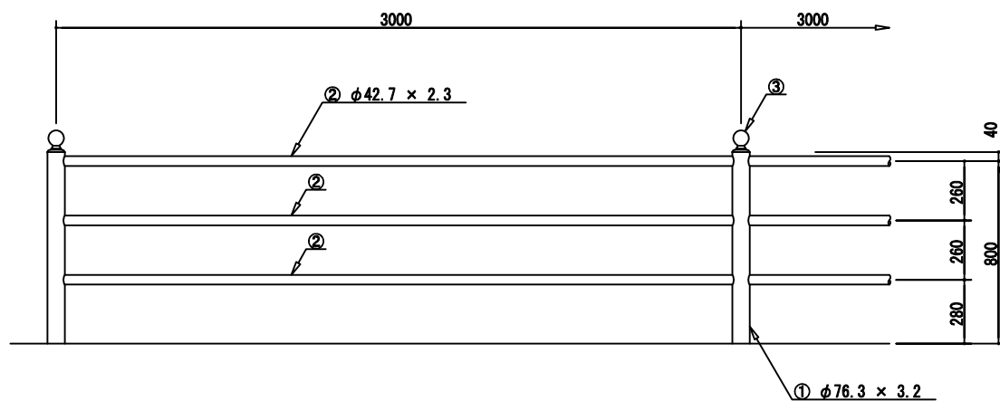
取付詳細図
