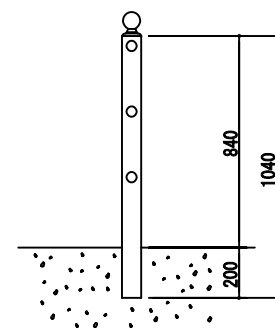
連続基礎式 (P7-308W)
