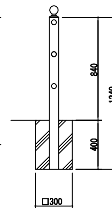
独立基礎式 (P7-308C)
