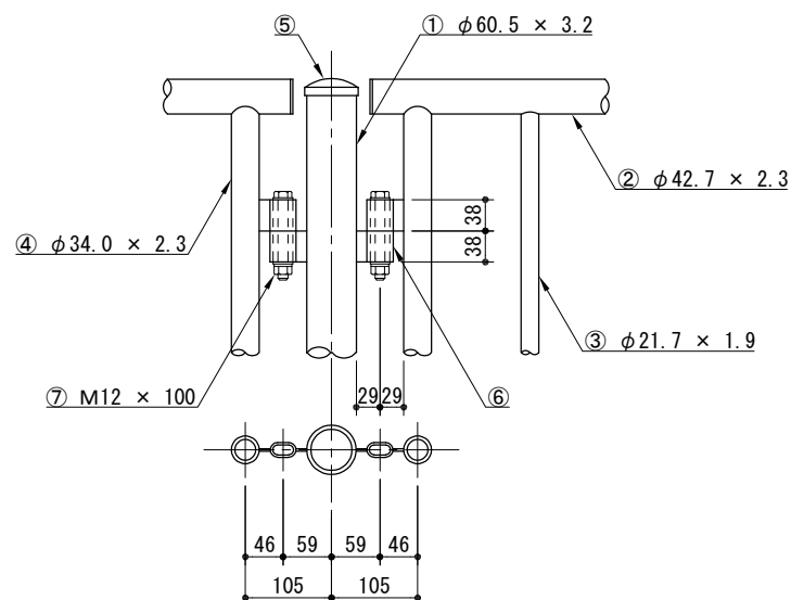
取付詳細図
