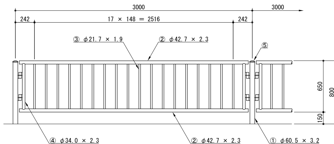
正面図
