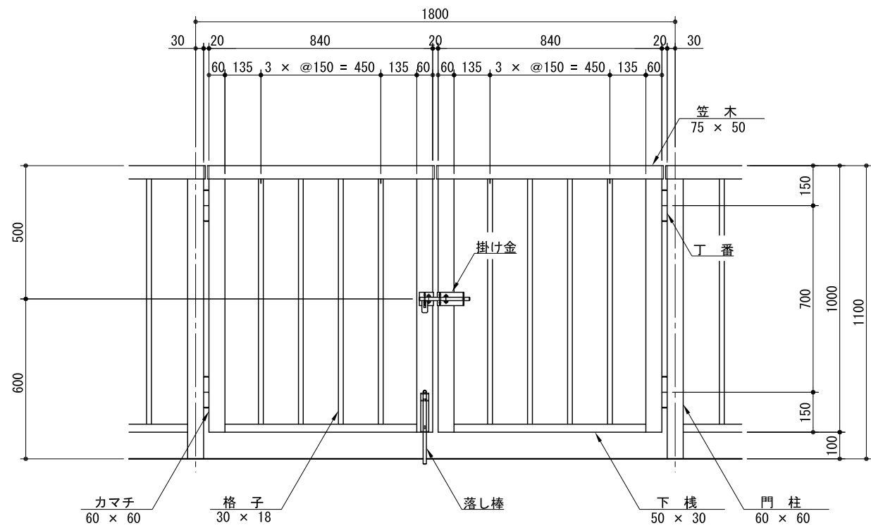
正面図
