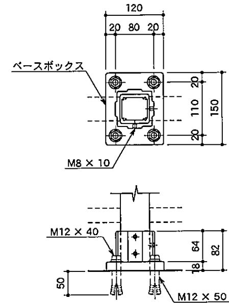
ベース部詳細図
