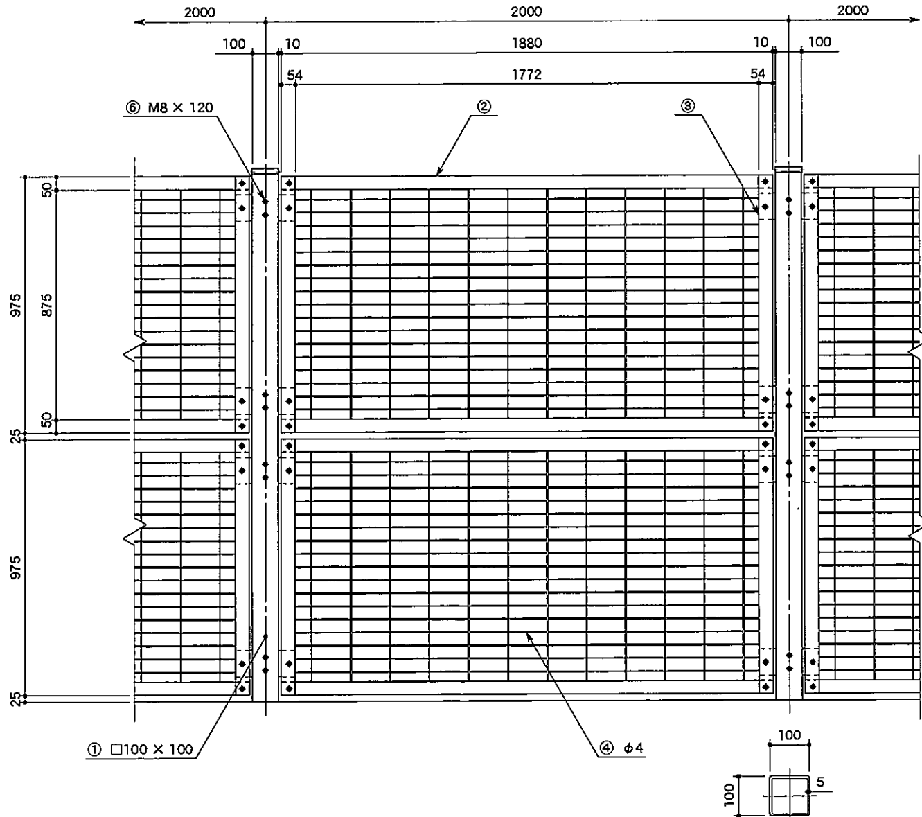
正面図
