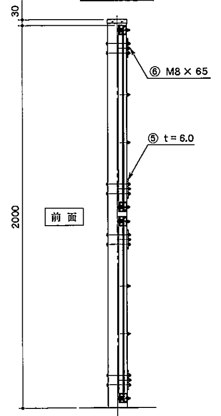
側面図
