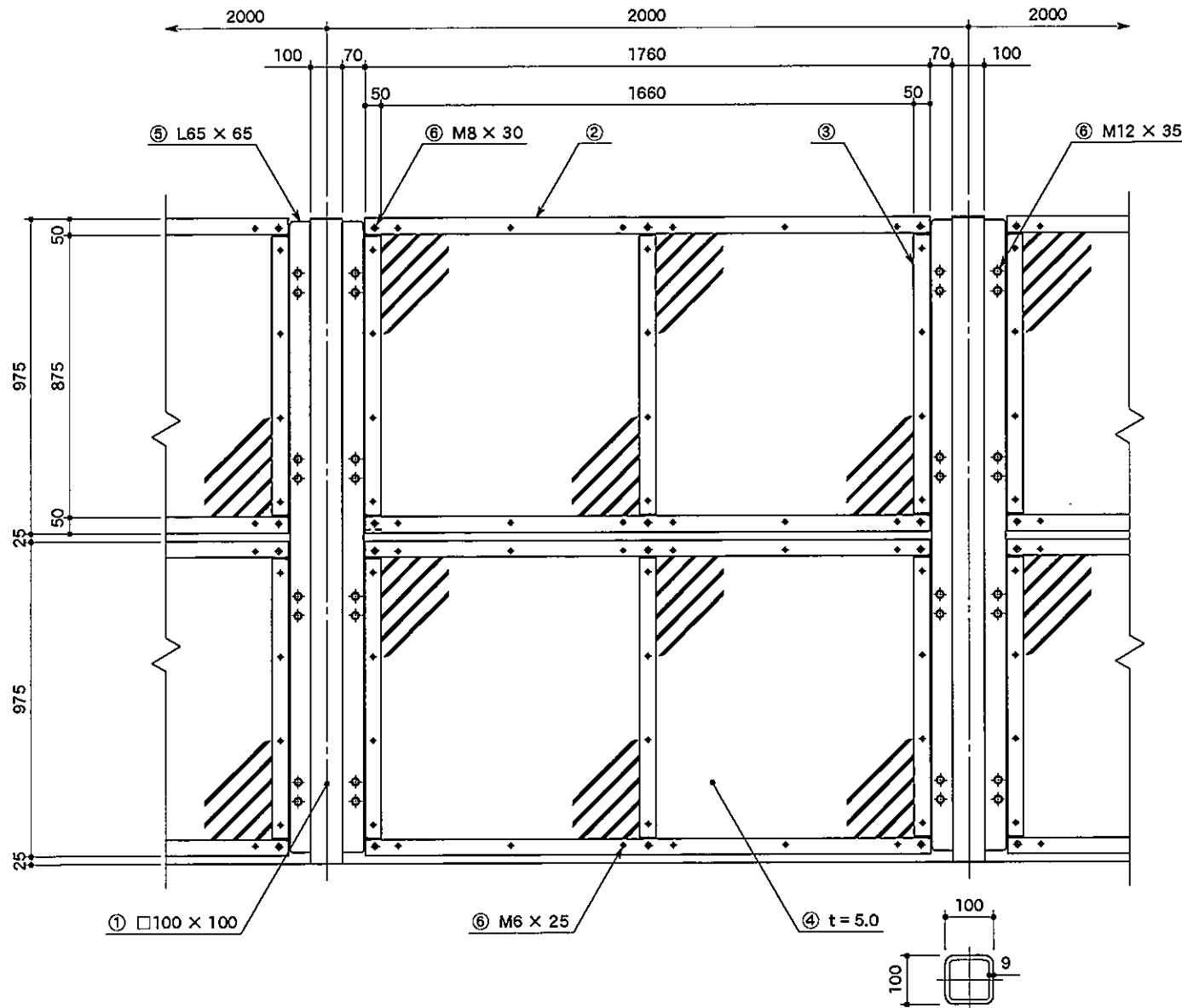
正面図
