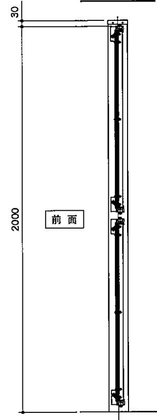
側面図
