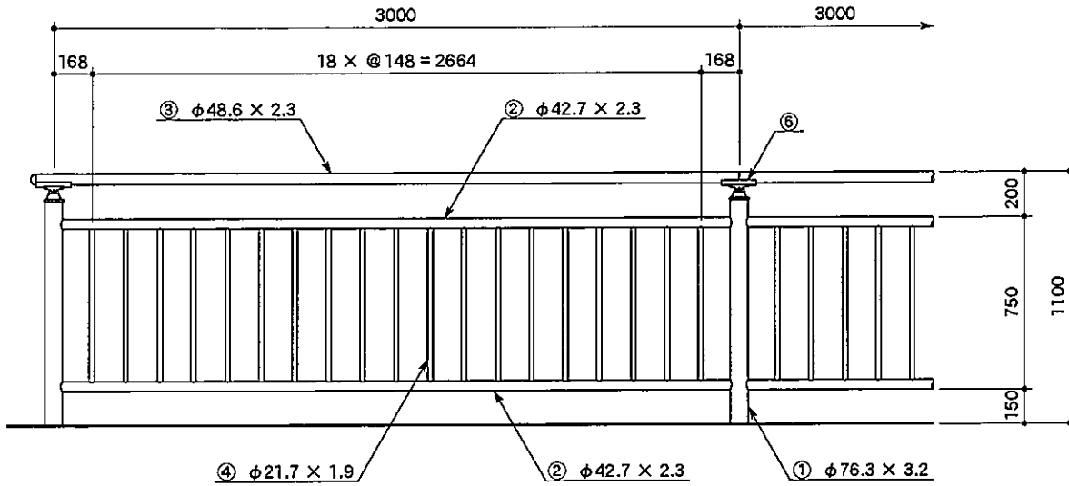
取付詳細図
