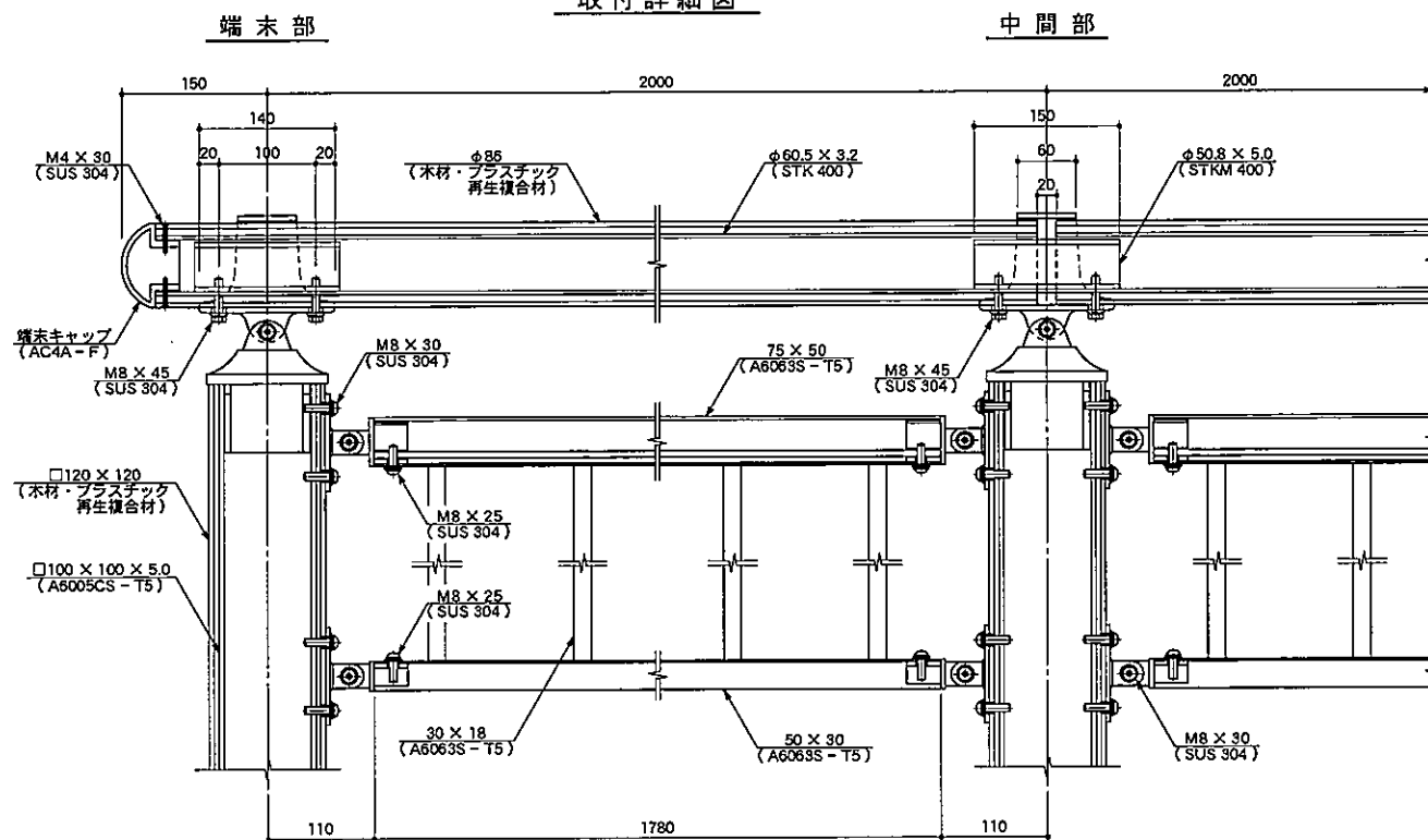
取付詳細図
