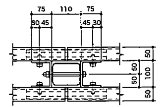
C-C断面
