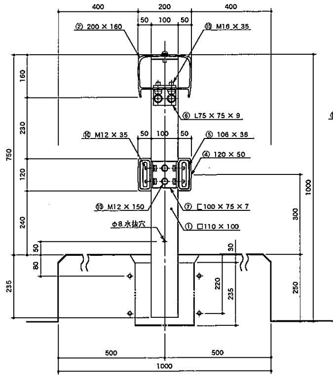
取付詳細図
