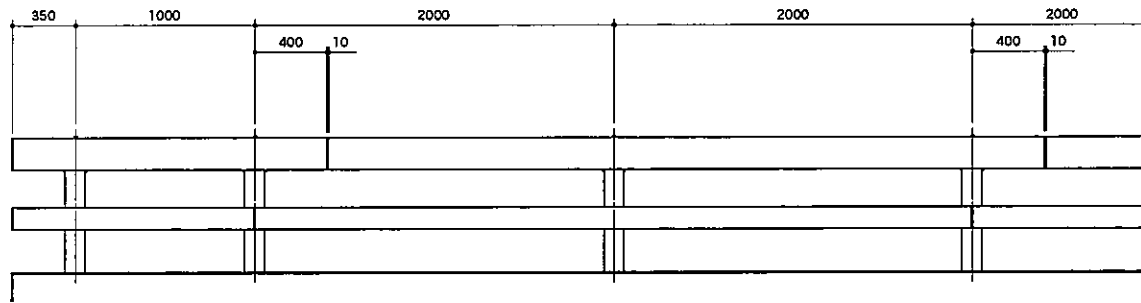
正面図
