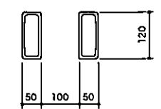
C-C断面
