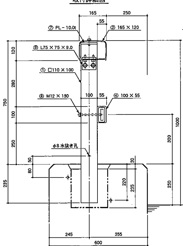
取付詳細図
