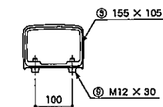
A-A 断面
