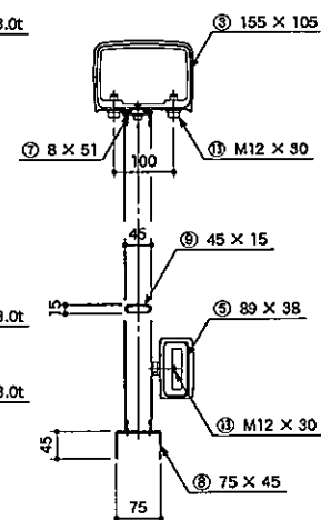
A-A 断面
