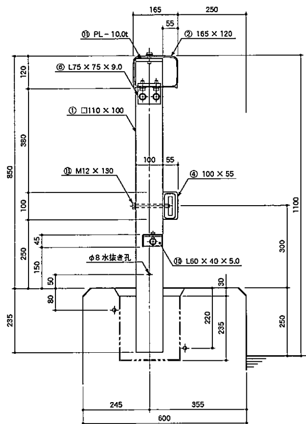
取付詳細図
