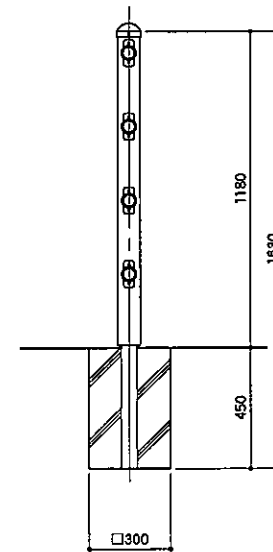
独立基礎式 (PEW-3-411C)
