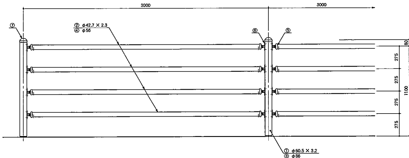
取付詳細図
