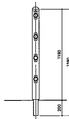
連続基礎式 (PEW-3-411W)
