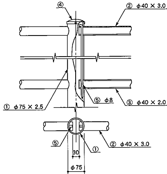
取付詳細図
